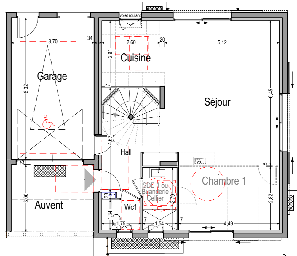
REZ DE CHAUSSEE - VILLA 5
