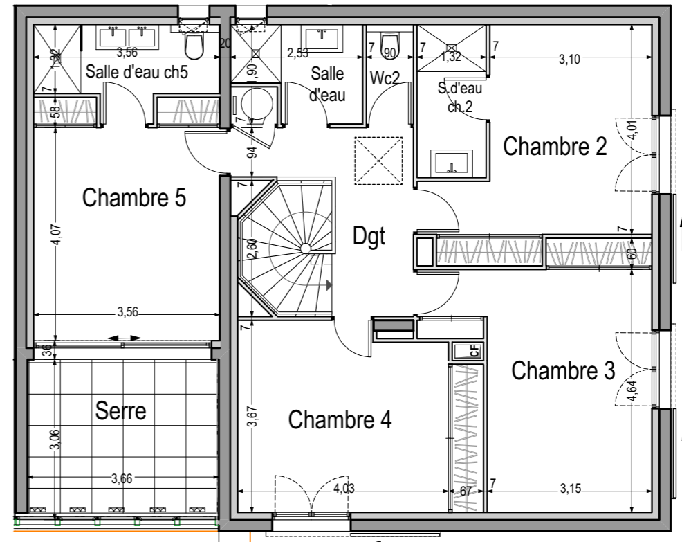
ETAGE - VILLA 5
