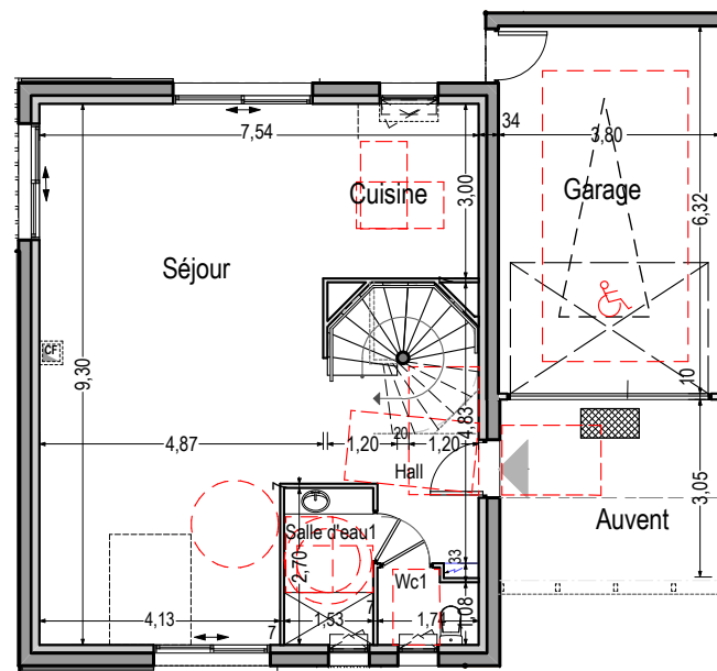
REZ DE CHAUSSEE - VILLA 4
