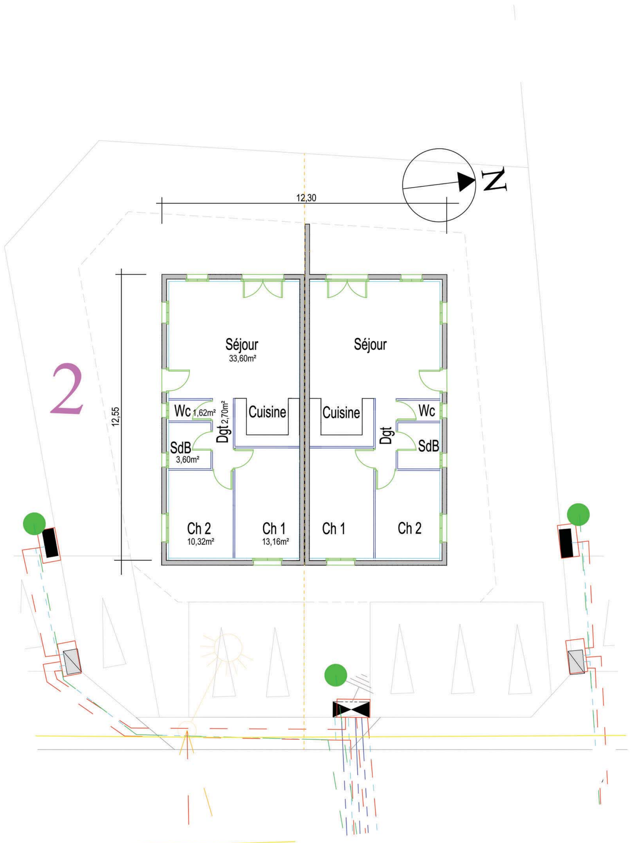
Villa à 2 logements (65m 2 par logement) "Les Coteaux de Campiergues" NEBIAN ECH : 1/100
